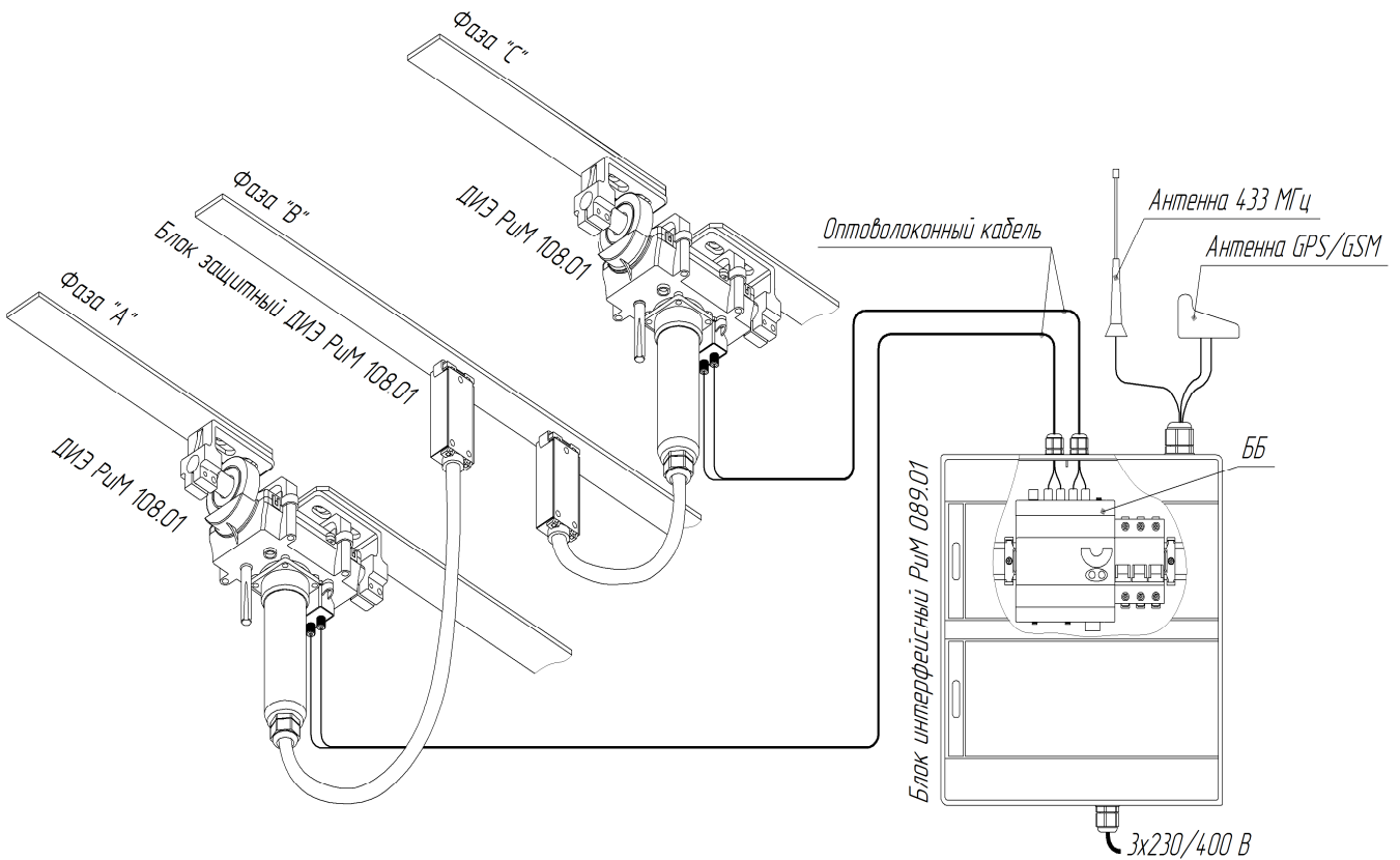
Рисунок 5 – Пример установленного ИПУЭ на ТП
