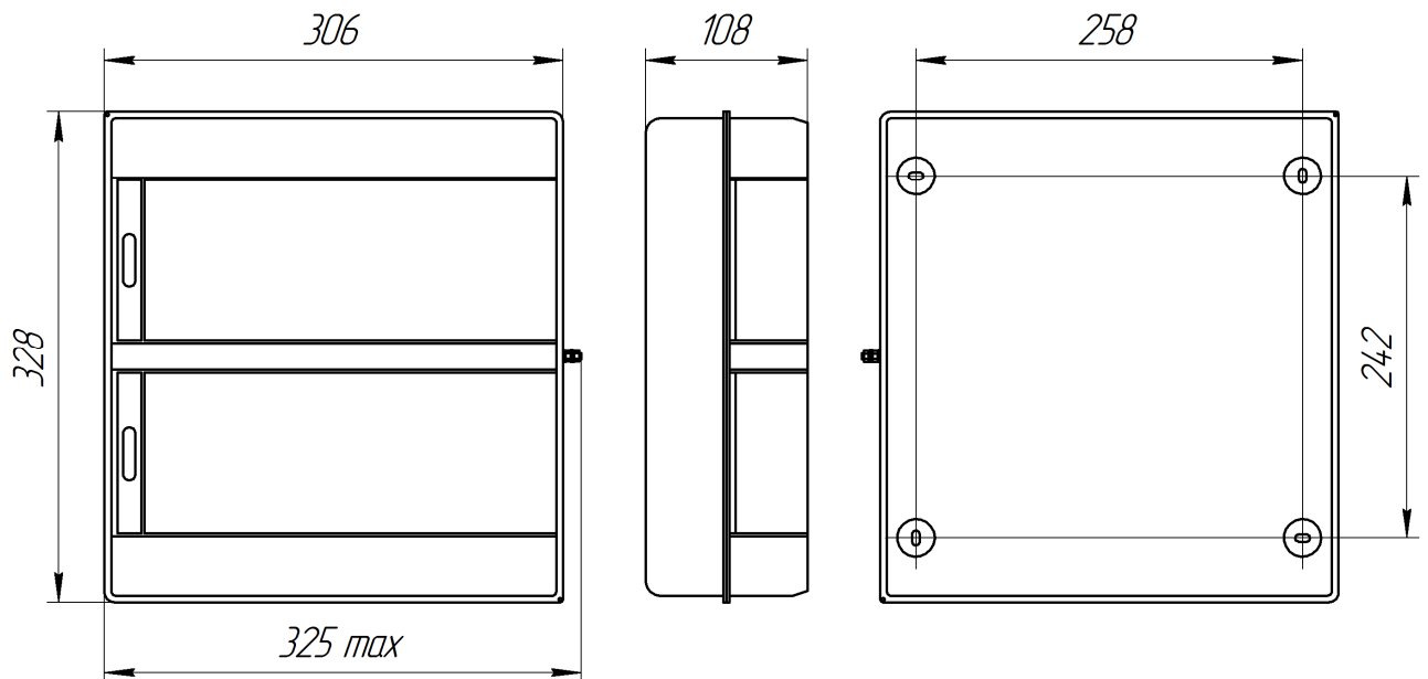
Рисунок 2 – Габаритные, установочные размеры ДИЭ
