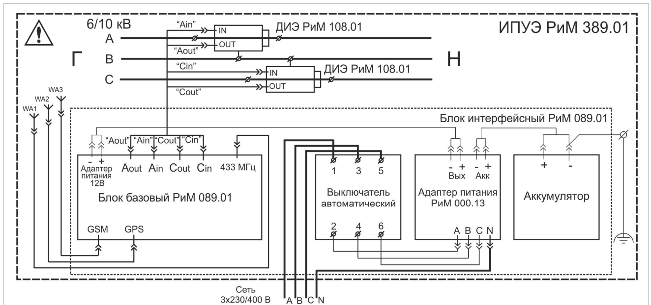
Рисунок 4 – Схема подключения ИПУЭ
